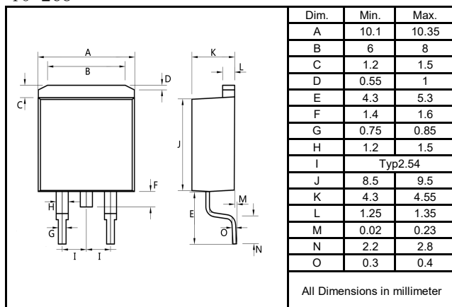
T0-263
